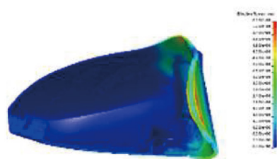
変形メカニズムイメージ (フェースセンター打点 H/S40m/s) 変形倍率10倍
